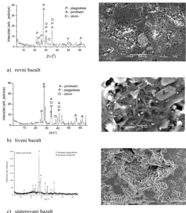
Slika 1. XRD difraktogram i SEM mikrofotografija uzorka rovnog bazalta (a) i staklo-keramike na bazi livenog i sinterovanog bazalta (b,c).
