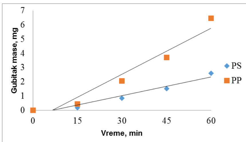
Slika 4. Kavitacione brzine uzorka premaza PP i PS.
